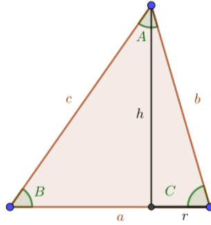
Figura 3.10: Triangle no rectangle i la seva altura perpendicular al costat a
