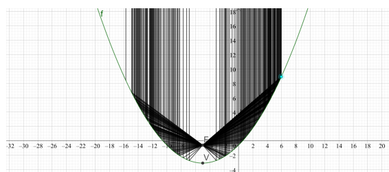
(b) Paràbola: les rectes perpendiculars a la directriu es reflecteixin de manera que totes es tallen al focus.
