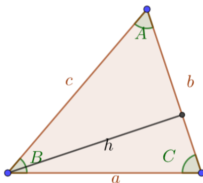
Figura 3.9: Triangle no rectangle i l'altura perpendicular a b .
