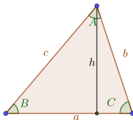
Figura 3.8: Triangle no rectangle i l'altura perpendicular a a .
