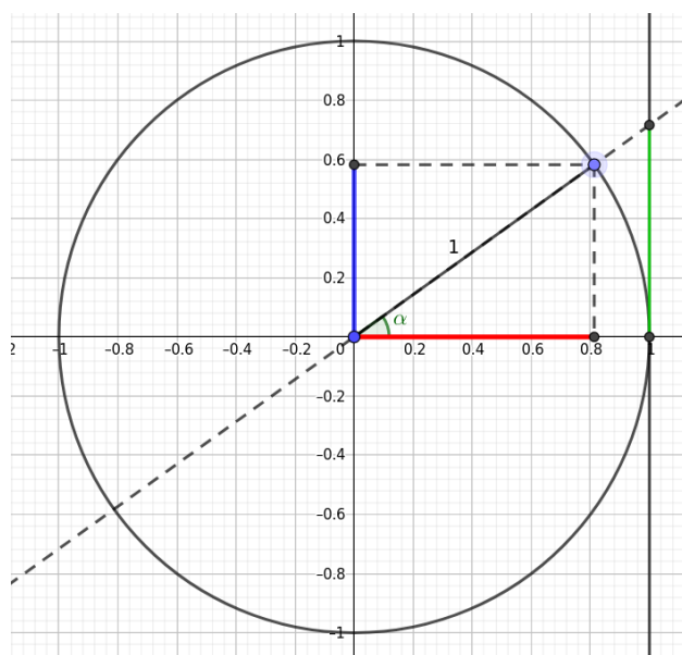
Figura 3.1: Sinus, cosinus i tangent d'un angle qualsevol.
